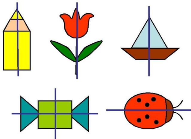
Симметричные фигуры
